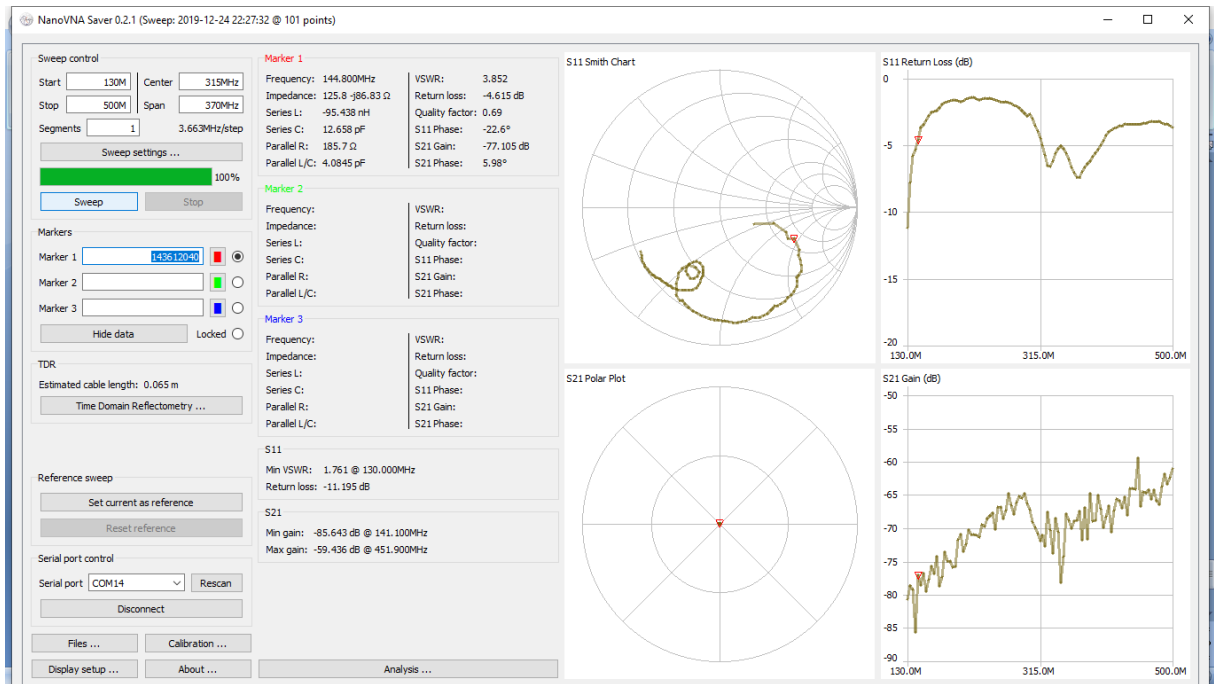
Lambda/4 pro 2m pline vysunuta
